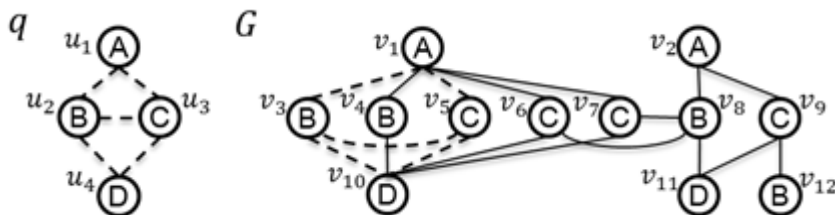
그림. Subgraph isomorphism의 예. 데이터 그래프 G 에서 쿼리 그래프 q 를 검색하면 \{(u_1, v_1), (u_2, v_3), (u_3, v_5), (u_4, v_{10})\} 이렇게 한 개의 embedding이 나온다(파선으로 표시).
